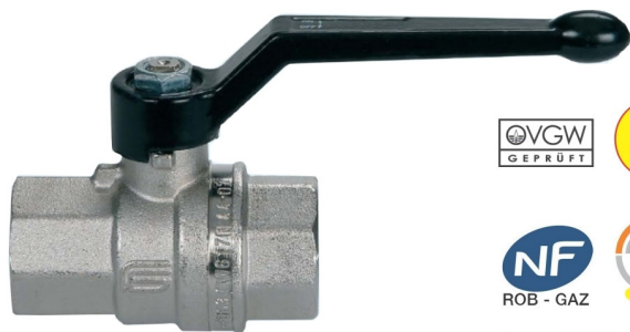
Art.1001 雙內牙 尺寸:1/4"-4" Art.1002 內外牙 尺寸:1/4"-2"1/2"
