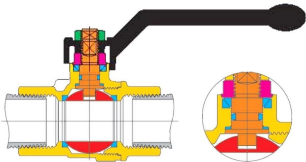
Art.1011 雙內牙 尺寸:1/4"-4" Art.1012 內外牙 尺寸:1/4"-2"1/2"
