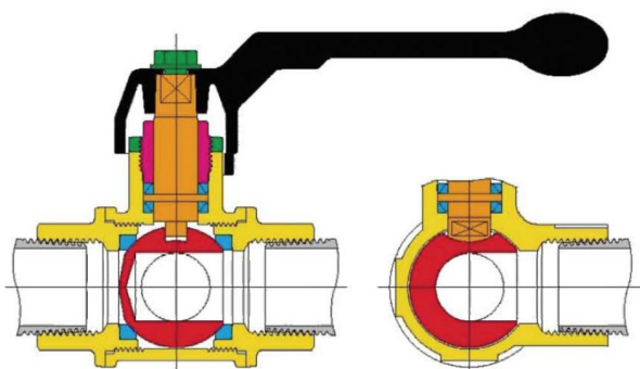
Art.1150 三通L型 尺寸:1/4"~2"
