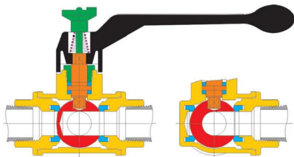
Art.1100 三通L型 尺寸:1/4"~2" Art.1120 三通T型 尺寸:1/4"~2"
